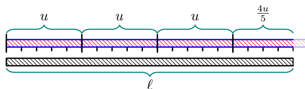
Figura 3.6: uma barra \ell que mede 19/5 unidades de comprimento.
