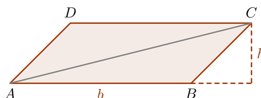
Figura 9.16: um paralelogramo de base b e altura h .
