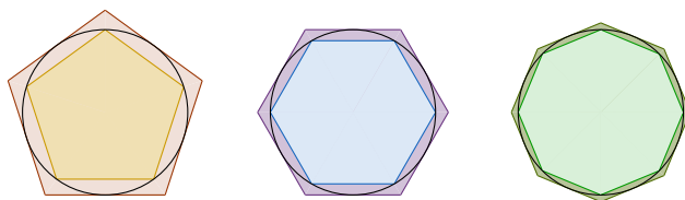
Figura 9.4: Arquimedes estimou a área do círculo pelo método da exaustão empregando polígonos regulares inscritos e circunscritos com uma quantidade arbitrariamente grande de lados. As figuras acima são “meramente ilustrativas” já que Arquimedes não partiu de pentágonos nem fez uso de octógonos. Ele começou com hexágonos regulares e prosseguiu dobrando a quantidade de lados dos polígonos que ia obtendo.
