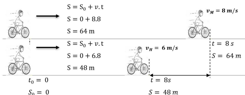
Figura 22– Representação de dois ciclistas
