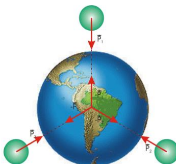
Figura 35. Força peso.
