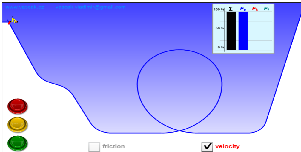
Figura 5. Print da simulação Conservação de Energia
