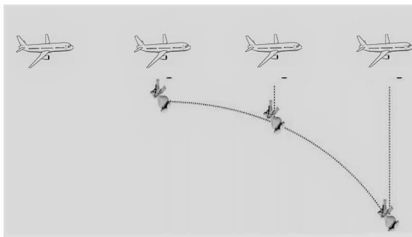
Figura 6- Trajetória do avião
