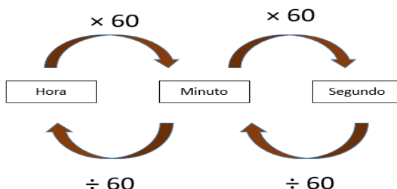
Figura 4- Conversão de tempo
