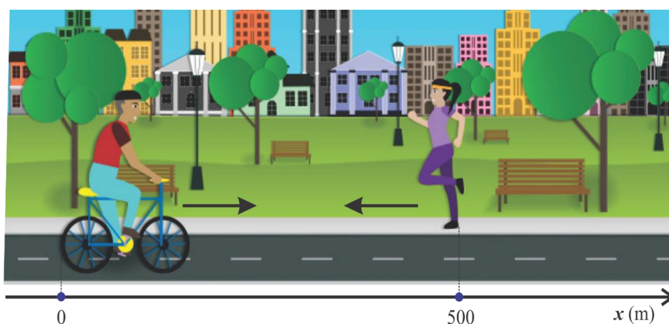
Figura 30- Encontro entre dois corpos, sentidos contrários
