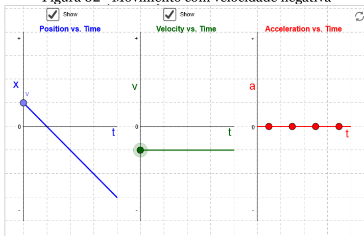
Figura 02 - Movimento com velocidade negativa
