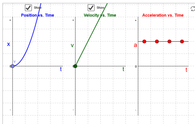
Figura 03 - Movimento com aceleração escalar positiva
