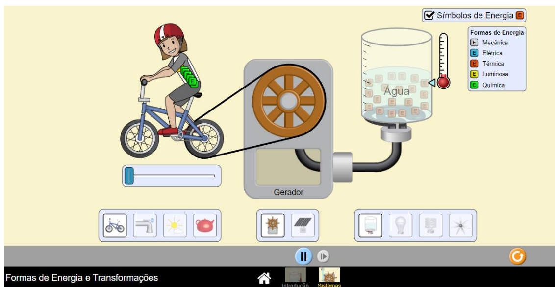
Figura 56 Print da simulação:
