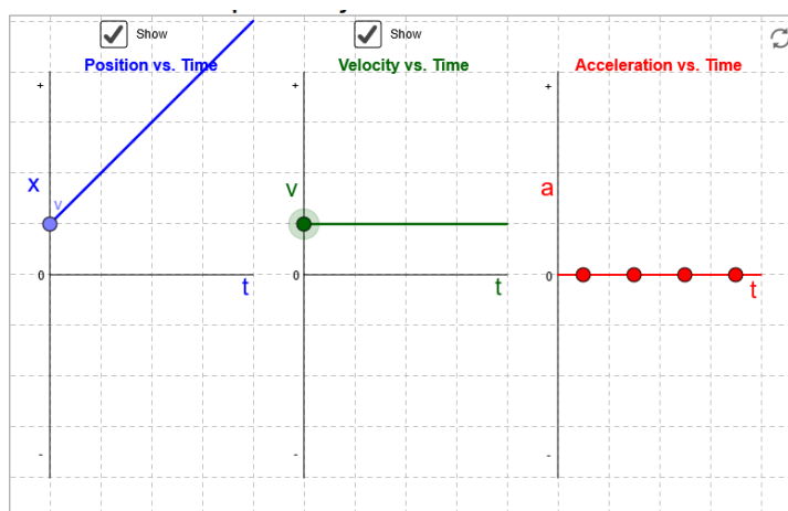
Figura 01 - Movimento com velocidade positiva
