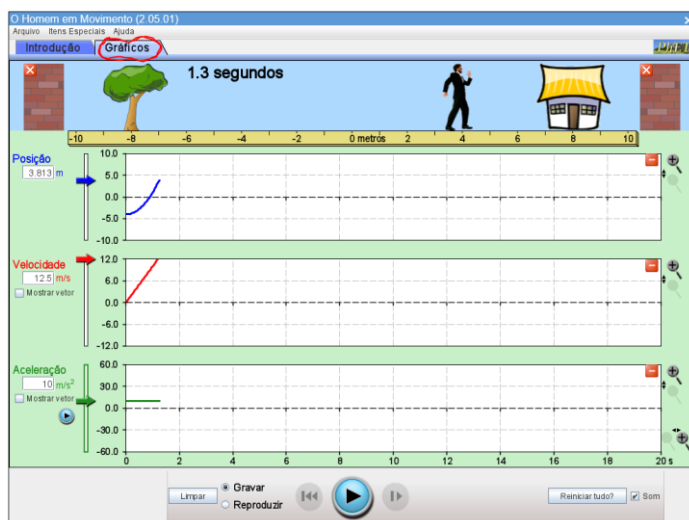
Figura 1 – Homem andando no sentido positivo da trajetória.
