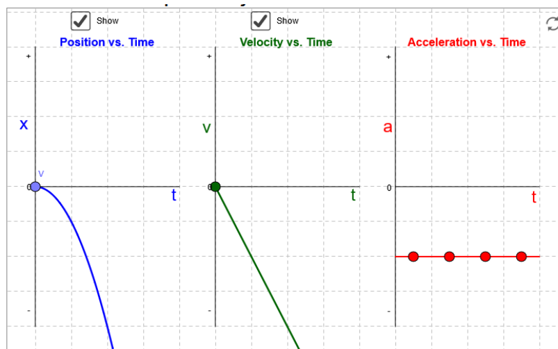
Figura 04 - Movimento com aceleração escalar negativa
