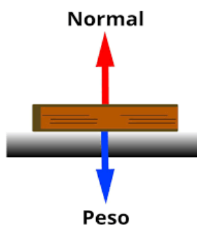
Figura 36. Forças atuando sobre o livro em uma superfície horizontal.
