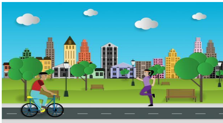
Figura 29- Encontro entre dois corpos
