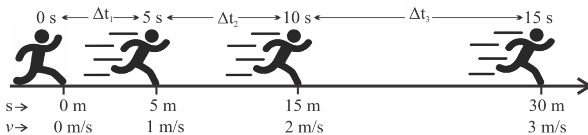
Figura 3 – Um corredor partindo da posição inicial 0 m e indo até uma posição final igual a 30 m no sentido positivo da trajetória.
