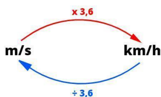
Figura 12- Conversão de unidades de velocidades
