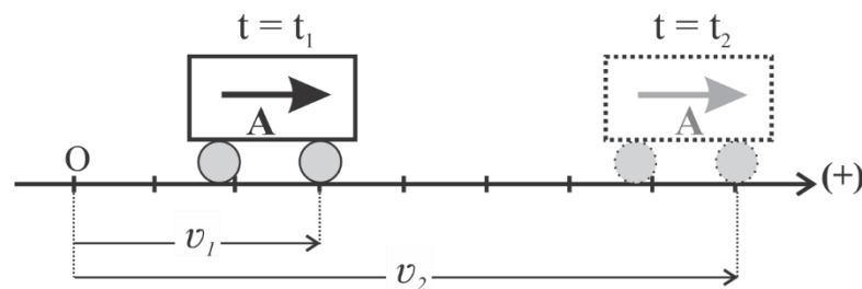
Figura 14- Carrinho A com velocidade inicial v_1 no tempo inicial t_1 e com velocidade final v_2 no tempo final t_2
