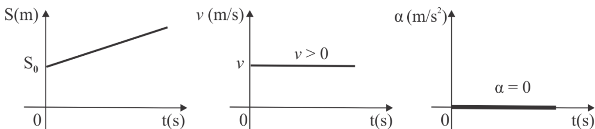
Figura 23- Movimento progressivo
