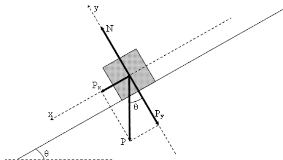
Figura 39. Plano inclinado.
