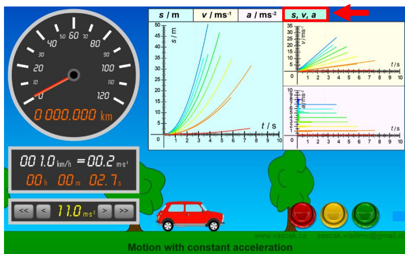
Figura 4 – Gráficos de simulações simultâneas da posição, velocidade e aceleração.
