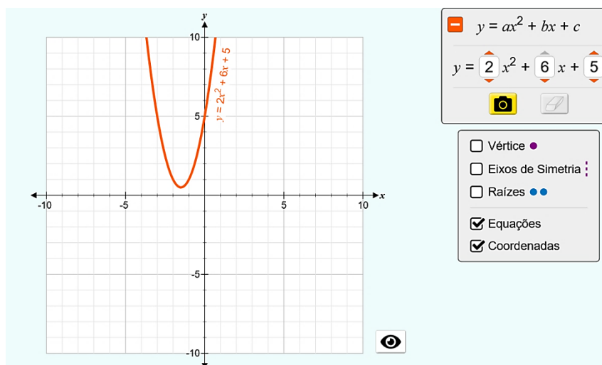
Figura 7 – Gráfico de uma função do 2º grau.
