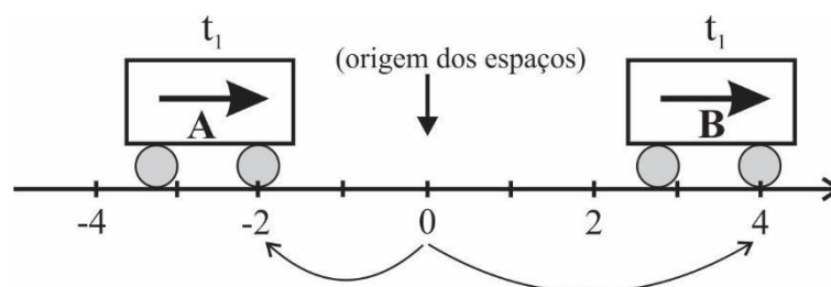
Figura 8 - Dois carrinhos distintos A e B em posições iniciais diferentes, em relação à origem dos espaços, ambos no mesmo instante de tempo
