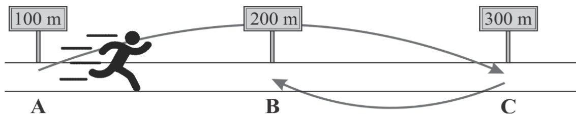
Figura 10- Corredor se deslocando ao longo de uma pista de corrida, indo do ponto A ao ponto C.
