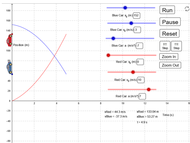
Figura 5 – Simulação gráfica de carros se movendo em sentidos opostos.
