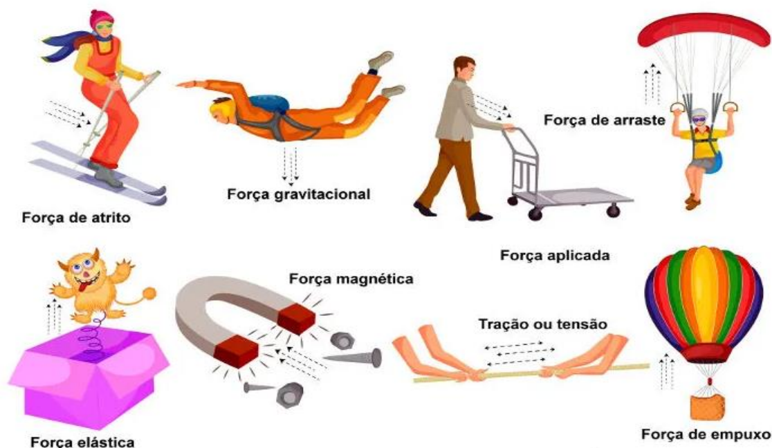
Figura 33. Existem diversos tipos de força.
