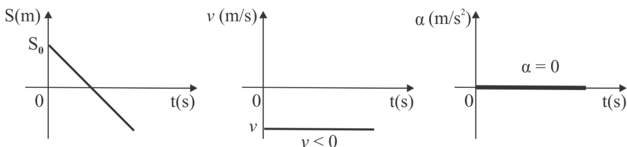
Figura 24- Movimento Retrógrado
