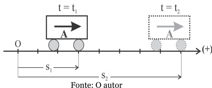
Figura 11- Carrinho A na posição inicial S_1 no tempo inicial t_1 e na posição final S_2 no tempo final t_2 .
