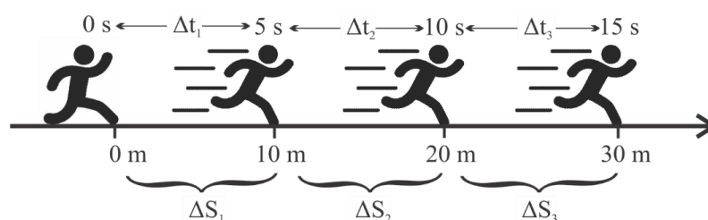
Figura 20- Um corredor partindo da posição inicial 0 m e indo até uma posição final igual a 30 m no sentido positivo da trajetória
